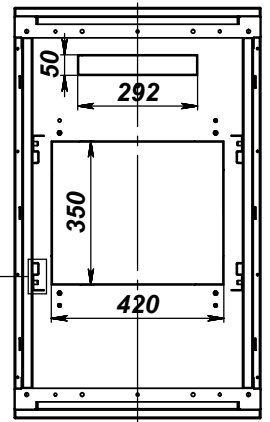
СЕЧЕНИЕ G-G МАСШТАБ 1 : 6.5
